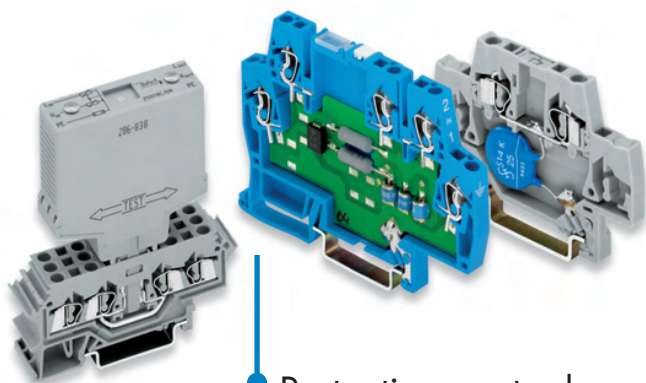
Protection contre les surtensions Overvoltage Protection 288 Series
